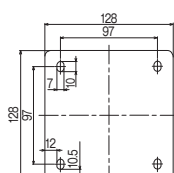
壁面設置金具 (穴寸法図)
