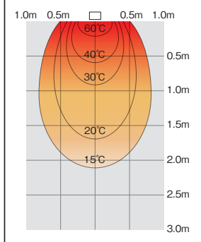
【温度分布図(周囲温度10℃)】
