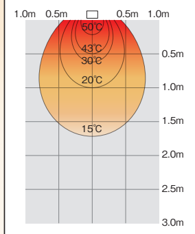
【温度分布図(周囲温度10℃)】
